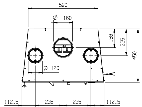
INSERTO 70 VENTILATO
